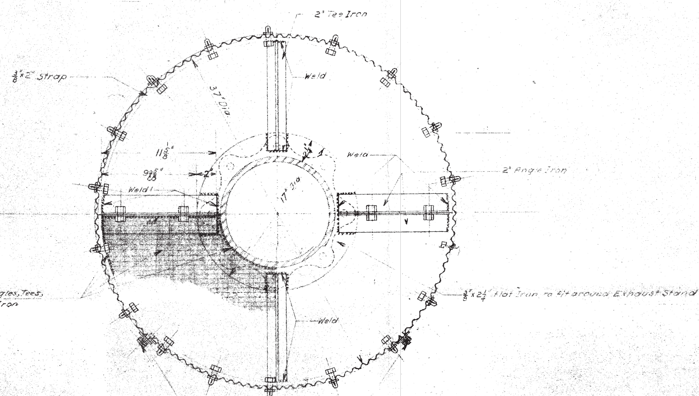
Section A-A
